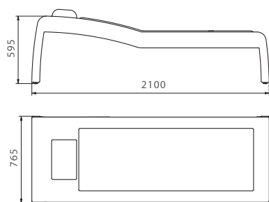
Dimensions Couchette Reina
