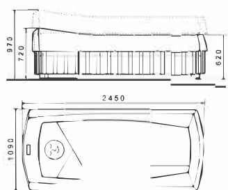
Toneca-Spa avec habillage design
