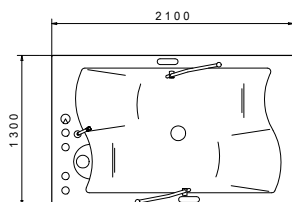
Dimensions de la «Rendela»
