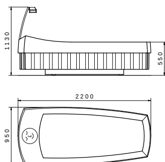
Dimensions AquaTonecajet
