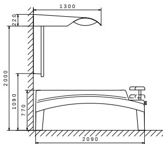
Dimensions Douche Arc-en-Ciel
