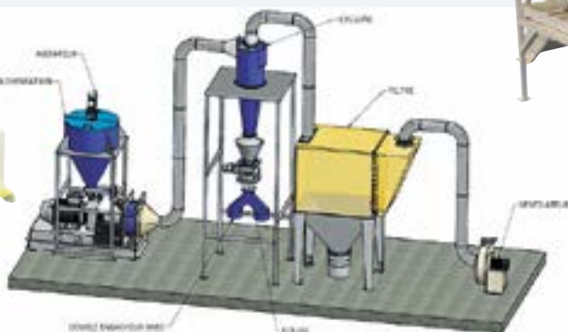
Unité de micronisation MIC4 30 kW
