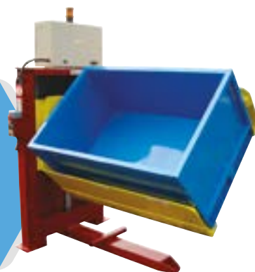
ÉLÉVATEUR INCLINEUR
